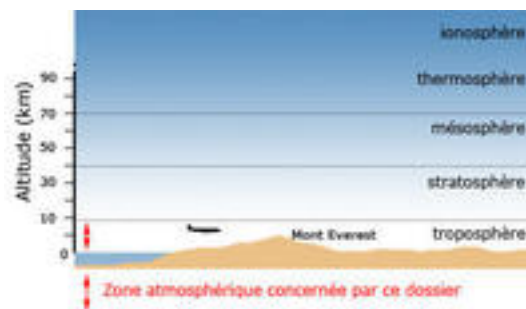
Coupe de l'atmosphère
